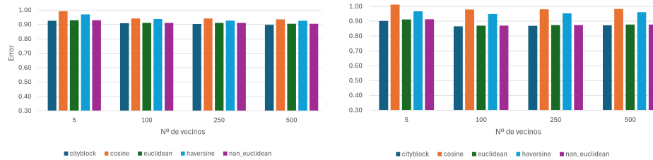
Fig. 2. Error medido por MAE en MovieLens para el experimento de aleatorización del sistema (izquierda) o de datos (derecha).
