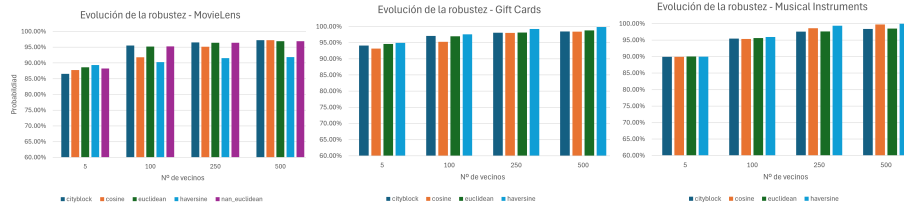
Fig. 1. Robustez frente a la aleatorización del sistema en MovieLens (izquierda), Gift Cards (medio) y Musical Instruments (derecha).
