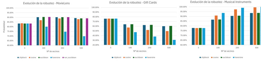
Fig. 3. Robustez frente a la aleatorización de los datos en MovieLens (izquierda), Gift Cards (medio) y Musical Instruments (derecha).
