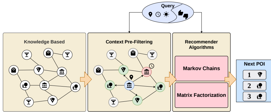
Figura 1. Esquema general del sistema de recomendación. Se estructura en 3 pasos: (1) modelado del dominio y del contexto en un grafo; (2) prefiltrado contextual; y (3) aplicación de modelos de recomendación.
