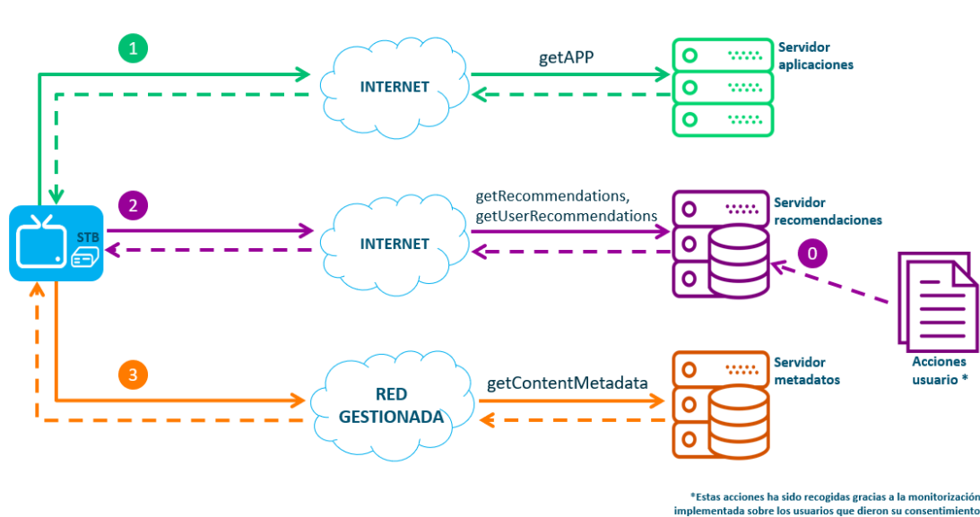
Figura 3.1: En esta figura se muestra la arquitectura que se construido para poder ofrecer las recomendaciones.
